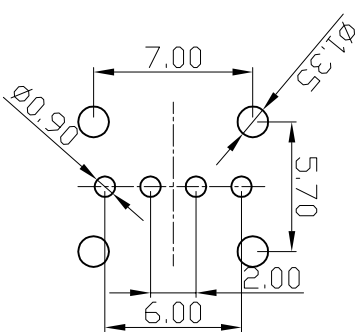
P.C.B LAYOUT (对接尺寸)
